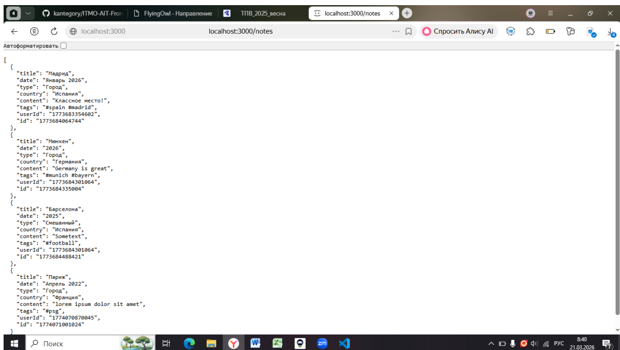
Рис.3. Данные о пользовательских заметках на сервере
